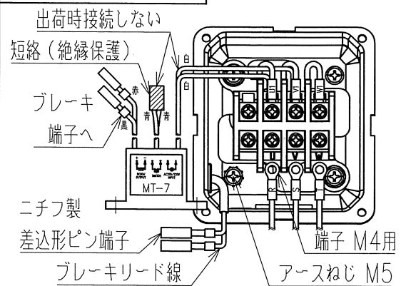
結線図（同時切りの場合）
