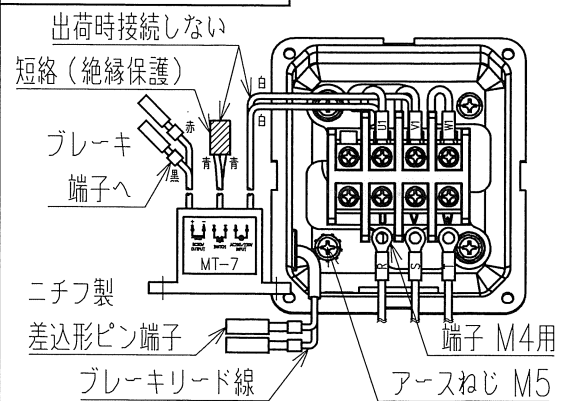
結線図（同時切りの場合） Not to scale
