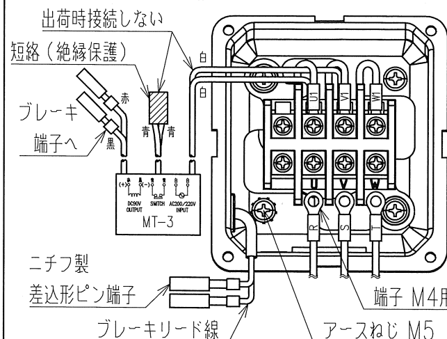
結線図（同時切りの場合）
